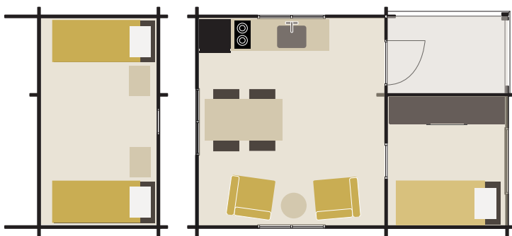
Månäs 25 + 10 kvm (6000x4150 mm, varav altan 2280x1530 mm) passar som sommarstuga, gäststuga eller bostad året runt. Stugan har takförsedd hörningång med altan och ett loft. Välj bland många tillbehör för att sätta din egen prägel.
